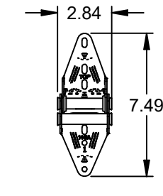
Edge Hinge .069 min. Galv. Steel (14 ga.)
